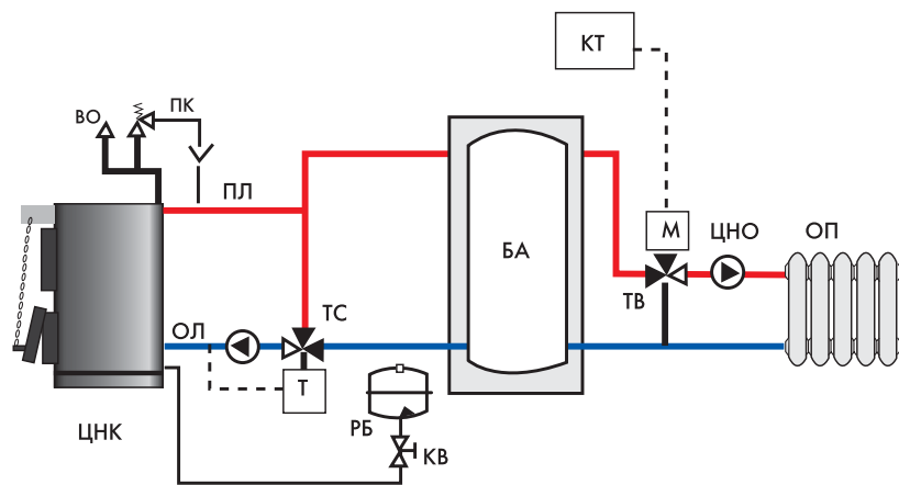
Рис. 6. Примерная схема обвязки твердотопливного котла с баком-аккумулятором: ПЛ – подающая линия; ОЛ – обратная линия; ПК – предохранительный клапан; ВО – автоматический воздухоотводчик; РБ – расширительный бак; КВ – колпачковый вентиль; ЦНК – циркуляционный насос котла; ТС – термостатический смеситель; ОП – отопительный прибор; БА – бак-аккумулятор; ТВ – трехходовой вентиль с приводом; КТ – комнатный термостат; ЦНО – циркуляционный насос отопления
