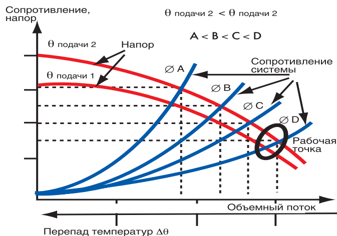
Рис. 3. Зависимость напора от разности температур при фиксированных температуре подачи и мощности котла в гравитационной системе отопления
