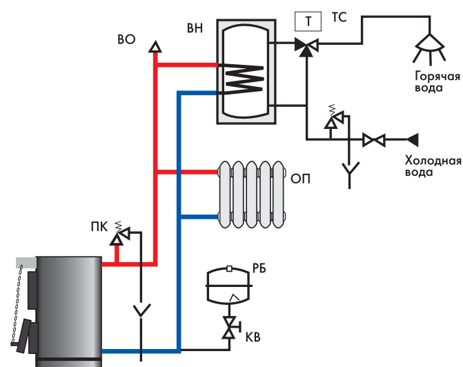
Рис. 2. Твердотопливный котел в гравитационной системе отопления с мембранным расширительным баком: ПК – предохранительный клапан; РБ – расширительный бак; КВ – колпачковый вентиль; ВО – автоматический воздухоотводчик; ТС – термостатический смеситель
